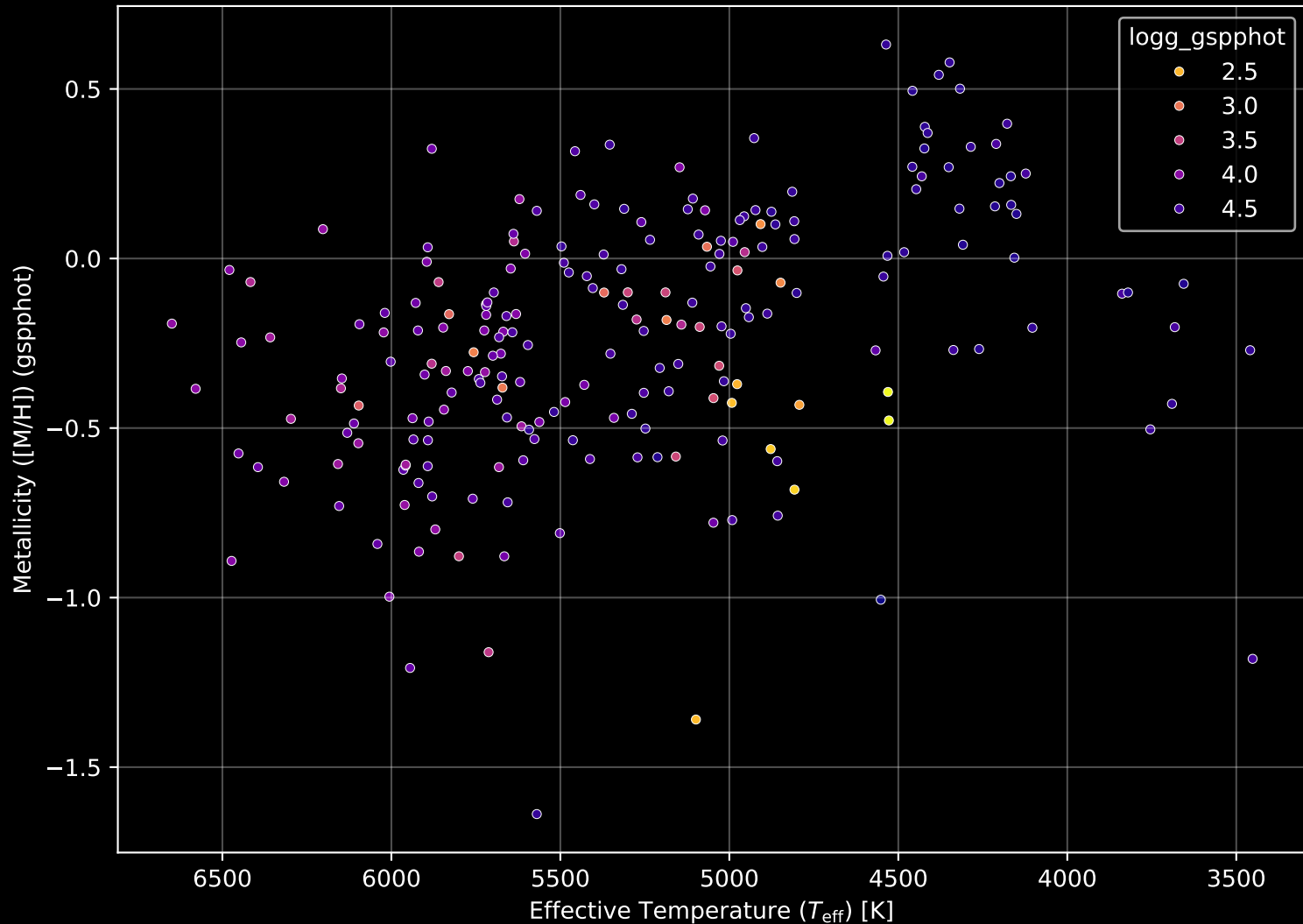
APOGEE DR17 Field: [272+58] Stellar Population Parameters (n= 222)
